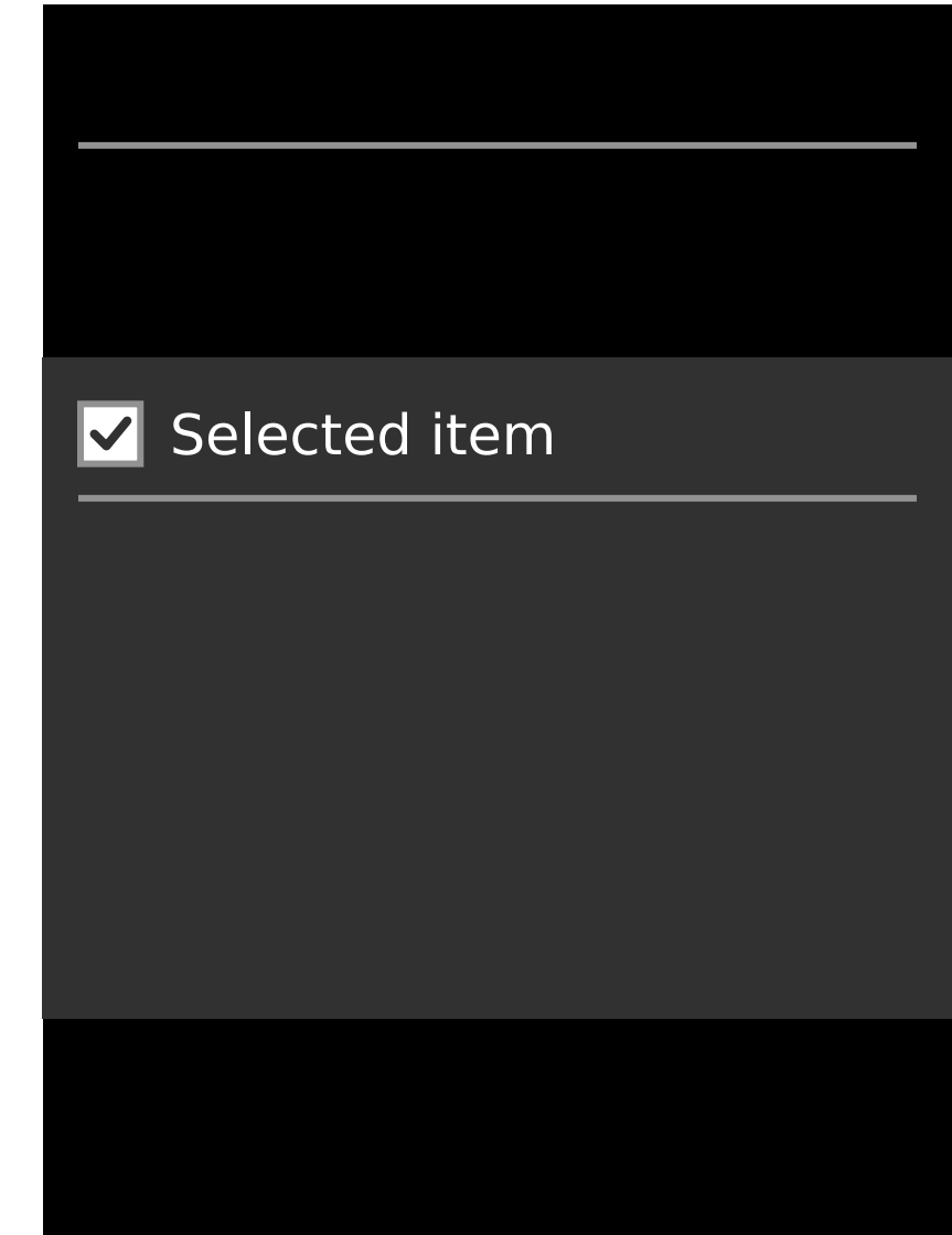
Checkbox
